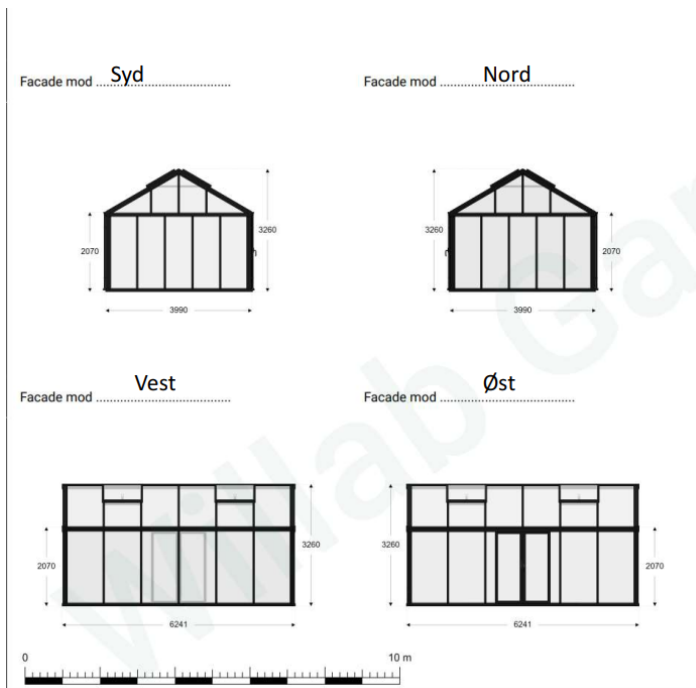
Figur 3 Udformning af drivhus
