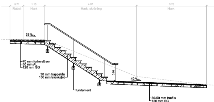
Figur 3. Udformning af trappeanlæg.
