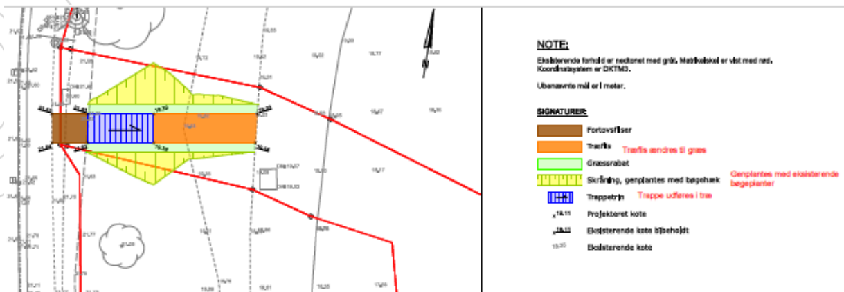
Figur 2. Placering af trappeanlæg.
