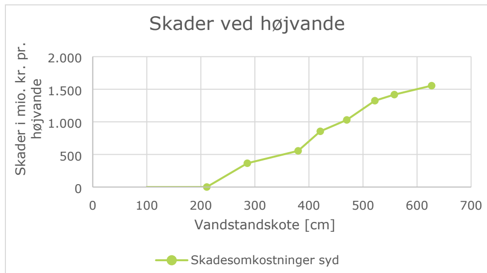
Figur 2-2 Skadesomkostningerne er gengivet som funktion af vandstandskoten. Disse stiger i takt med vandstanden, da flere ejendomme og anlæg bliver skadet.
