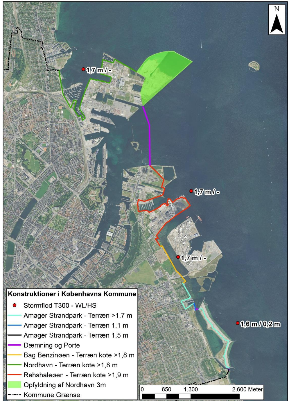
Figur 8-2 Stormflodskoten langs kysten ved en 300-års hændelse fra nord ved fire lokaliteter langs kysten. Bølgehøjden ved terrænet er angivet, hvor stormflodskoten overskrider det eksisterende terræn. Det eksisterende terræn angivet ved mulige konstruktioner langs Københavns Kommunes kyst. Det eksisterende terræn er lavere end stormflod ved to lokaliteter ved Amager Strandpark, hvor bølgehøjden kan have en effekt på terrænet. Forholdene for dæmninger og porte er angivet i Tabel 8-1.
