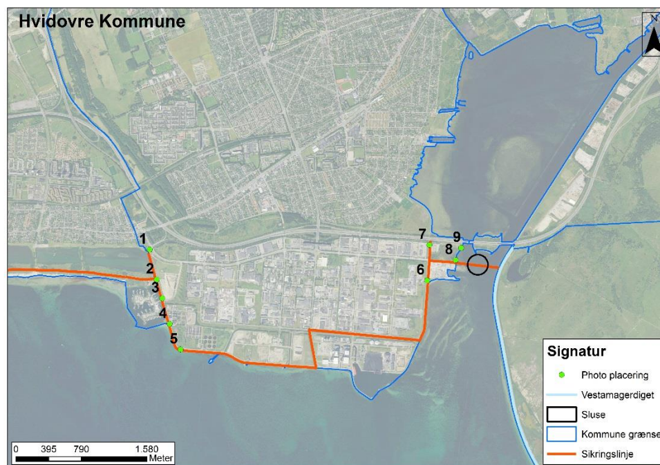
Figur 6-1 Oversigtskort med lokaliteter for fotos. På kortet er vist nuværende sikringslinje omkring Avedøre Holme samt placering af mulig sluse ved indløbet til Københavns Havn. Herved sikres de mest udsatte områder i København og Hvidovre kommuner mod stormflod fra syd.
