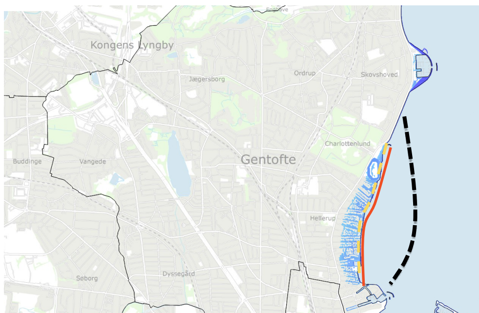
Figur 9-1 Illustration af de arealer der er mest udsat for oversvømmelser og skitsering af mulige sikringstyper for Gentofte. Gul stilet: sikring af enkeltejendomme, rød: gennemgående sikring, sort: gennemgående sikring i vandet. (SCALGOlive).
